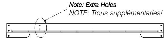
Front Stretcher (with extra holes) Rail d'étirement du devant (avec des trous en plus) x 1
