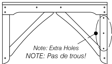
Lower End Frame (Right Hand) Pied de lit du bas (Côte droit) x 1
